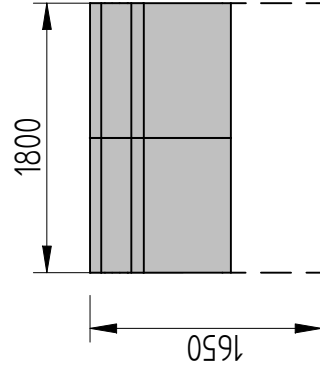
R2/1800 NI-21
