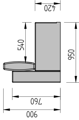
PODRŮČKA "B" POLOHOVATEĽNÁ SA-5250
