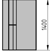
DVOJSED SEDADLO PEVNÉ HD-4/1400
