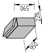
PODRUČKA "B" POLOHOVATEĽNÁ S NIKOU SA-6/250
