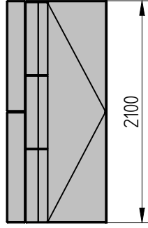
TROJSED SEDADLO ROZKLADACIE HD-2/2100
