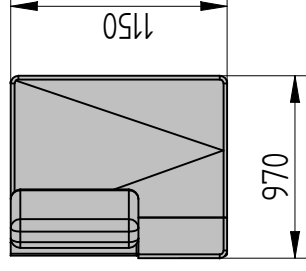
VÝKLOPNÁ ČASŤ MC-1/1150
