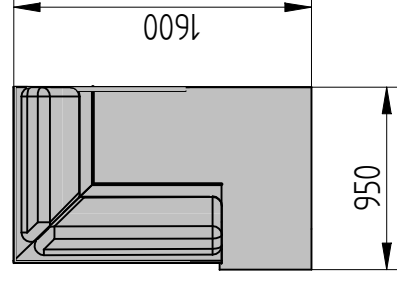
ROHOVÁ ČASŤ VÝKLOPNÁ MC-8/1600
